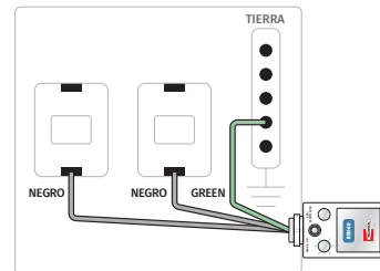
DIAGRAMA DE DESCONEXIÓN BIPOLAR DE 240 VCA
