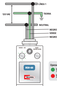
DIAGRAMA 120 VCA Sistema monofásico: 1 F, 2W + G
