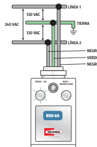
DIAGRAMA 240 VCA Sistema de fase dividida: 1 F, 2W + G
