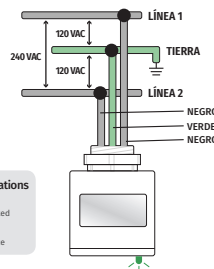
DIAGRAMA 240 VCA Sistema de fase dividida: 1 F, 2W + G
