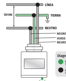
DIAGRAMA 120 VAC Sistema monofásico: 1 F, 2W + G
