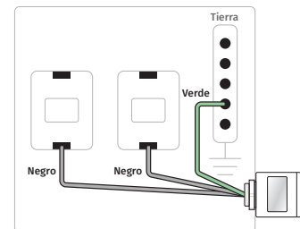
DESCONECTADOR BIPOLAR 240 VCA
