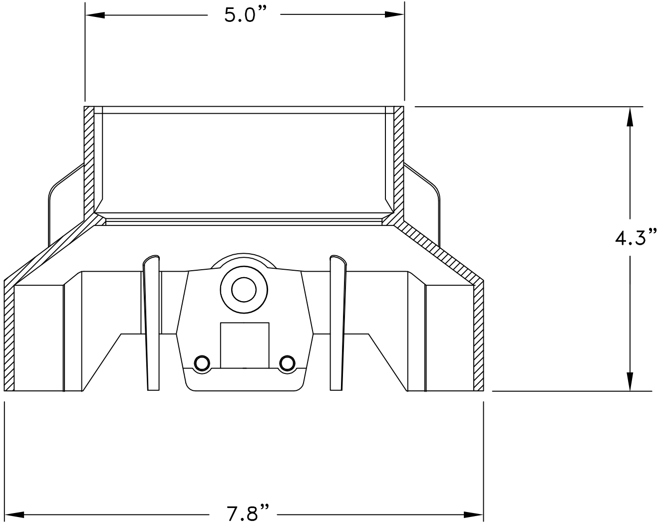
6" Upper/Lower Collar
